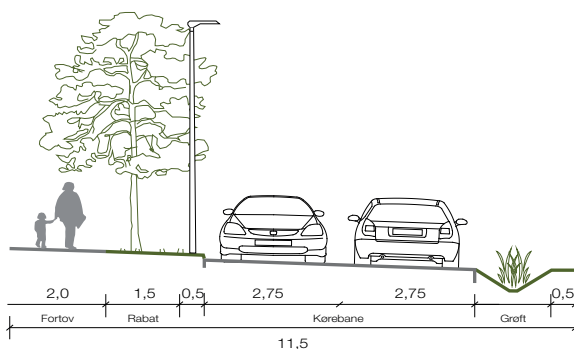
Illustration 1 Principiel tværprofil for boligvejen A.
